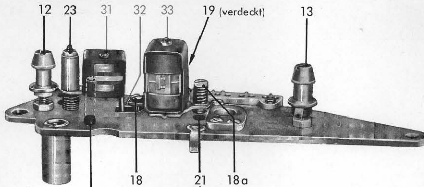
Bolzen für den Umlenkhebel (zur besseren Übersicht entfernt)
