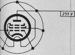
Rö. 3 EL 95
