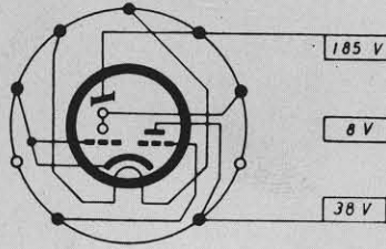
Rö. 4 EM 84
