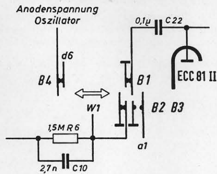
Kontaktanordnung und Verdrahtung
