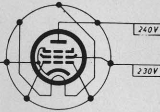
Rö. 5 EL 95
